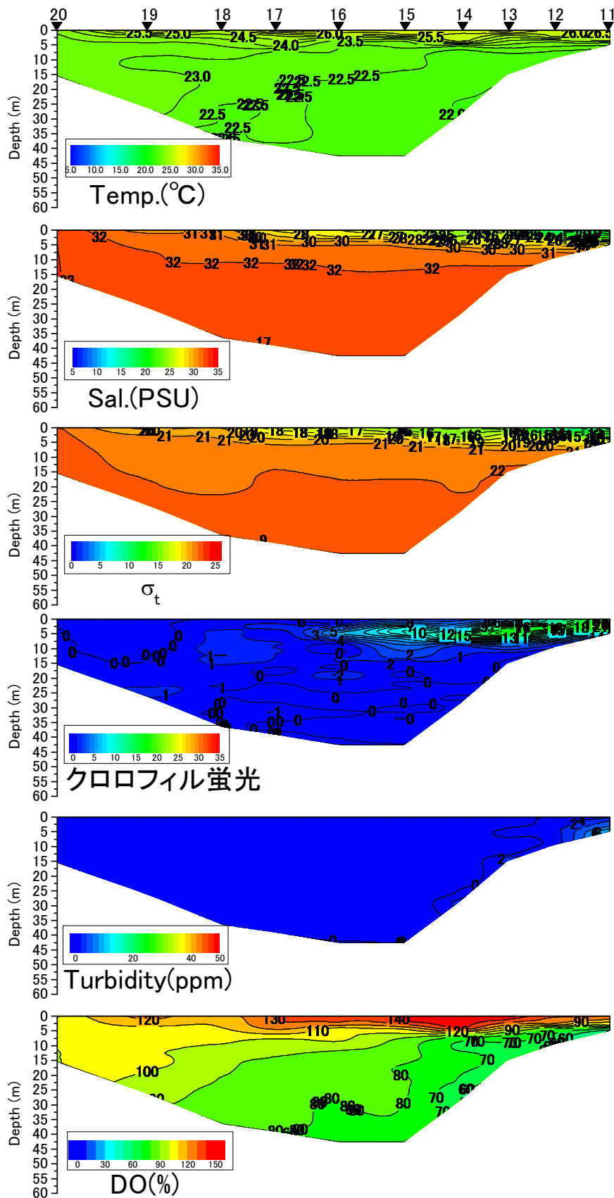
八代海中央ラインの水温(°C)、塩分、密度( \sigma_t )、クロロフィル蛍光強度、濁度、溶存酸素飽和度(DO%)の鉛直面図(国土交通省の調査による) (2014年7月18日)
