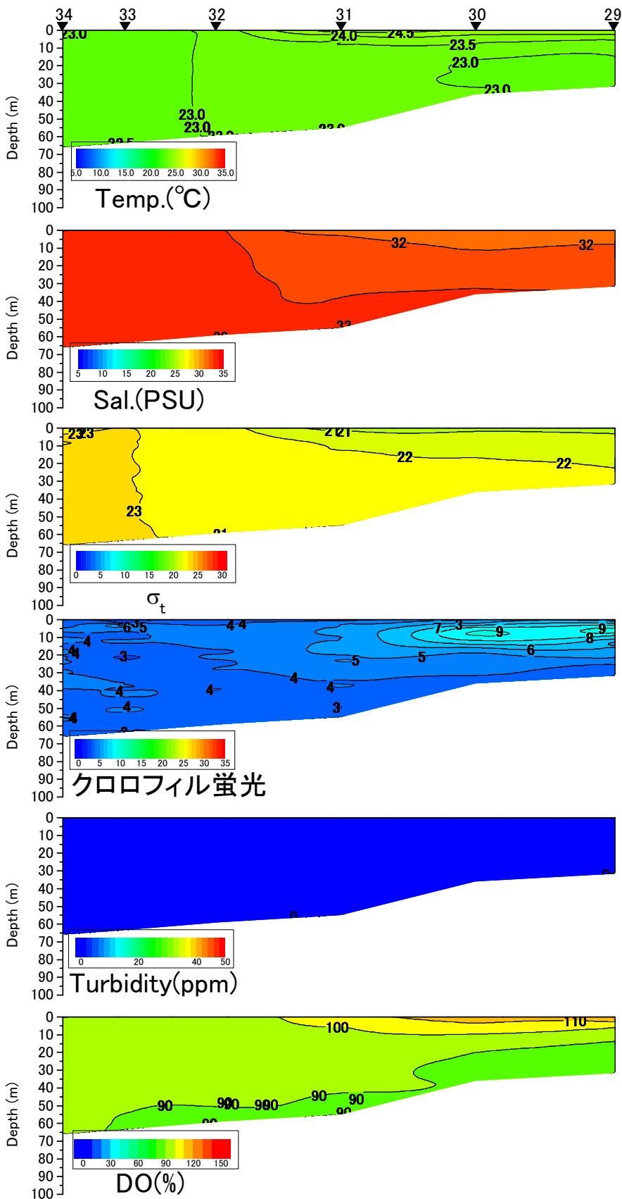
八代海西ラインの水温(°C)、塩分、密度( \sigma_t )、クロロフィル蛍光強度、濁度、溶存酸素飽和度(DO%)の鉛直面図(国土交通省の調査による) (2014年7月18日)
